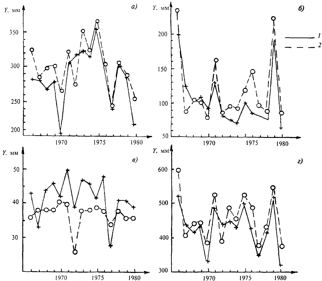
а) — весеннее половодье; б) — летне-осенний сезон; в) — сезон зимней межени; з) — годовое стока Рисунок А.5 — Сравнение фактических (1) и рассчитанных (2) слоев стока р. Вага — с. Усть-Сюма
