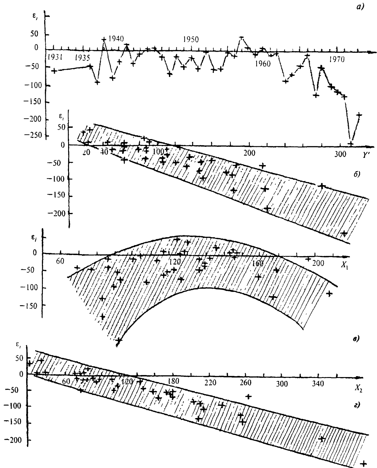
а) — зависимость остатков от времени ( \varepsilon = f(t) ); б) — зависимость остатков от значений слоя стока, полученного по эмпирической зависимости ( \varepsilon = f(Y') ); в) — зависимость остатков от первого фактора ( \varepsilon = f(X_1) ); г) — зависимость остатков от второго фактора ( \varepsilon = f(X_2) )
